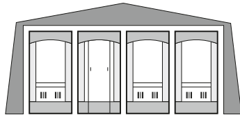
Voorwand (v. l. n. r.): Standaard raamsegment + hoog oprolbaar deursegment + standaard raamsegment + standaard raamsegment (v.a. maat: 18, 6 delig plus 2 standaard raamsegmenten)
